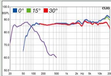
Geradliniger Frequenzverlauf ab ca. 80 Hertz selbst unter Winkel. Für ultimativen Tiefbass bis 25 Hertz sorgt der Sub P-10 DSS.
