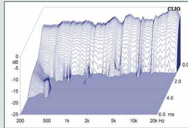
„SMC“ Technik im Magnetsystem und hochwertiger Hochtöner: es sind praktisch keine Resonanzen zu erkennen.
